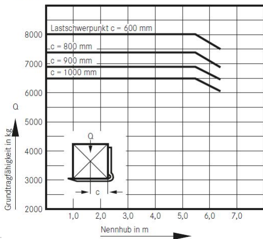
Grundtragungsfähigkeiten R 70-80
